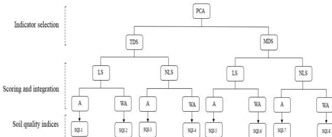
شکل ۲. نمودار فرآیند توسعه شاخص‌های کیفیت خاک. PCA: تجزیه به مؤلفه‌های اصلی، TDS: مجموعه کامل داده‌ها، MDS: مجموعه حداقل داده‌ها، LS: نمره‌دهی خطی، NLS: نمره‌دهی غیرخطی، A: روش ساده، WA: روش وزنی، SQI: شاخص کیفیت خاک.
