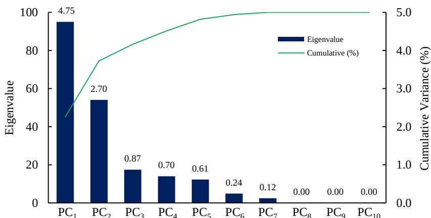
شکل ۳. تغییرات مقادیر ویژه مؤلفه‌های اصلی
