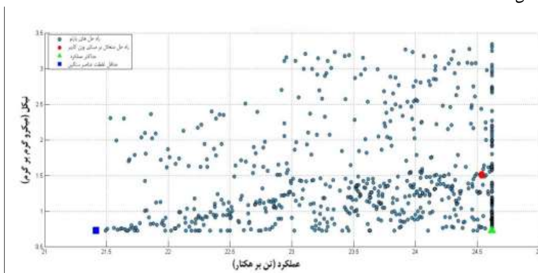
شکل ۳. راه‌حل‌های پارتو (Pareto Solution) و جبهه پارتو نهایی برای اهداف عملکرد و غلظت نیکل
