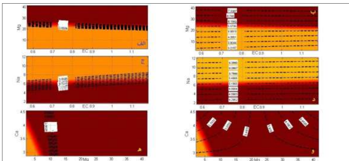
شکل ۵. سطوح پاسخ چندهدفه: اندرکنش پارامترهای کیفیت آب بر عملکرد (رنگ) و غلظت فلزات سنگین (خطوط هم‌مقدار). (الف) اثر متقابل EC و Mg بر عملکرد و نیکل. (ب) اثر متقابل EC و Mg بر عملکرد و کادمیم. (پ) اثر متقابل EC و Na بر عملکرد و نیکل. (ت) اثر متقابل EC و Na بر عملکرد و کادمیم. (ث) اثر متقابل Ca و Mg بر عملکرد و نیکل. (ج) اثر متقابل Ca و Mg بر عملکرد و کادمیم.
