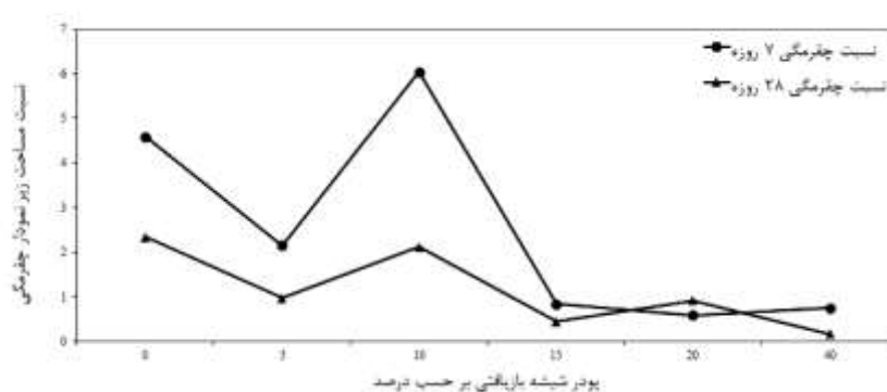
شکل ۵. نمودار تغییرات نسبت چقرمگی نمونه‌های ۷ و ۲۸ روز قبل از مقاومت حداکثر به بعد از آن بر حسب درصد‌های مختلف ژئوپلیمر
