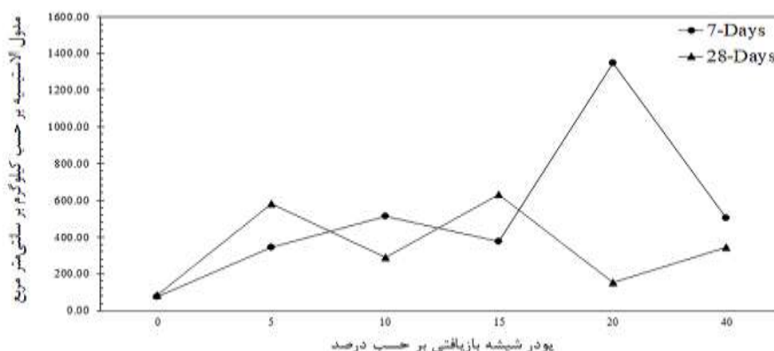
شکل ۸. نمودار تغییرات مدول الاستیسیته در مقابل درصد ژئوپلیمر بر پایه پودر شیشه بازیافتی
