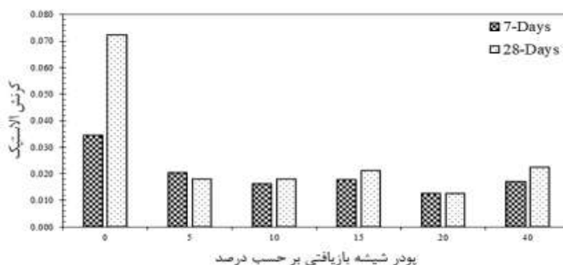
شکل ۷. نمودار تغییرات کرنش الاستیک در مقابل درصد افزودنی ژئوپلیمر
