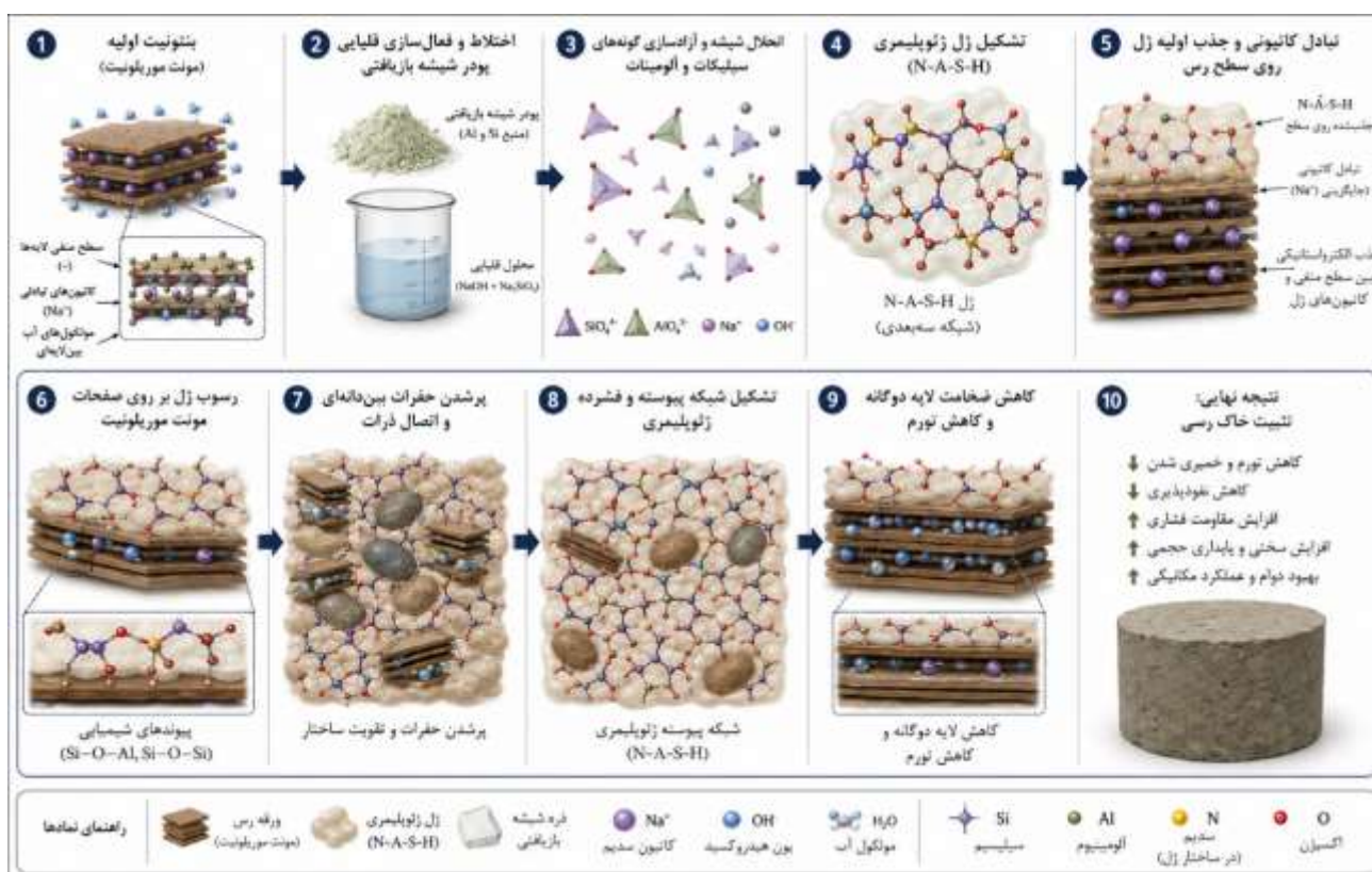
شکل ۲. شماتیک مکانیزم تثبیت بنتونیت حاوی مونت موریلونیت با ژئوپلیمر بر پایه پودر شیشه بازیافتی و جانشینی ژئوپلیمر بر روی سطح دانه‌های رسی
