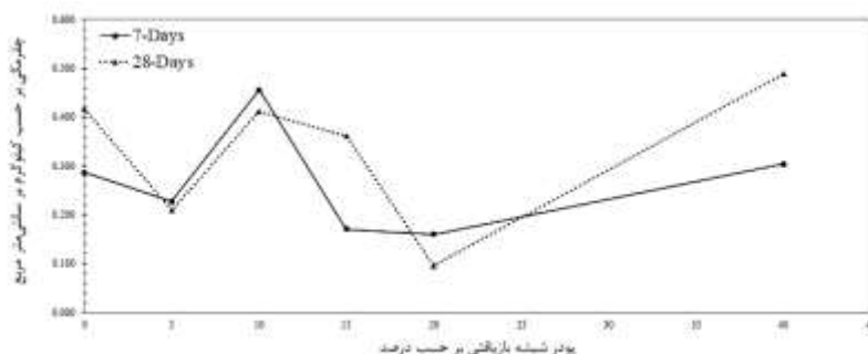
شکل ۶. نمودار تغییرات چقرمگی در مقابل درصد افزودنی ژئوپلیمر
