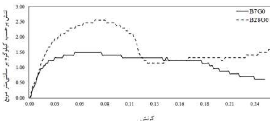
شکل ۳. نمودار تنش-کرنش نمونه های ۷ و ۲۸ روز بنتونیت تثبیت نشده
