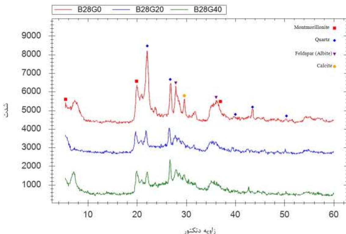
شکل ۱۰. نمودار پراش بر توی اشعه ایکس نمونه بنتونیت ۷ روز تثبیت شده با ۲۰ درصد ژئوپلیمر بر پایه پودر شیشه بازیافتی
