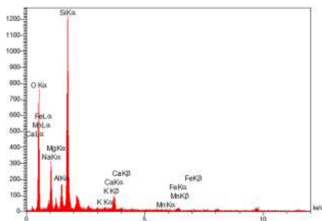
(الف) نمودار پراکندگی عناصر
