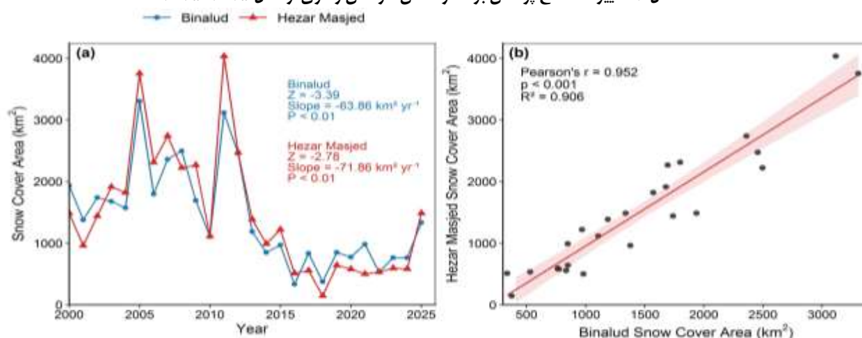
شکل ۴. تغییرات سطح پوشش برف (a) و همبستگی بین سطح پوشش برف سالانه (b) در ارتفاعات هزار مسجد و بینالود طی دوره ۲۰۲۵-۲۰۰۰
