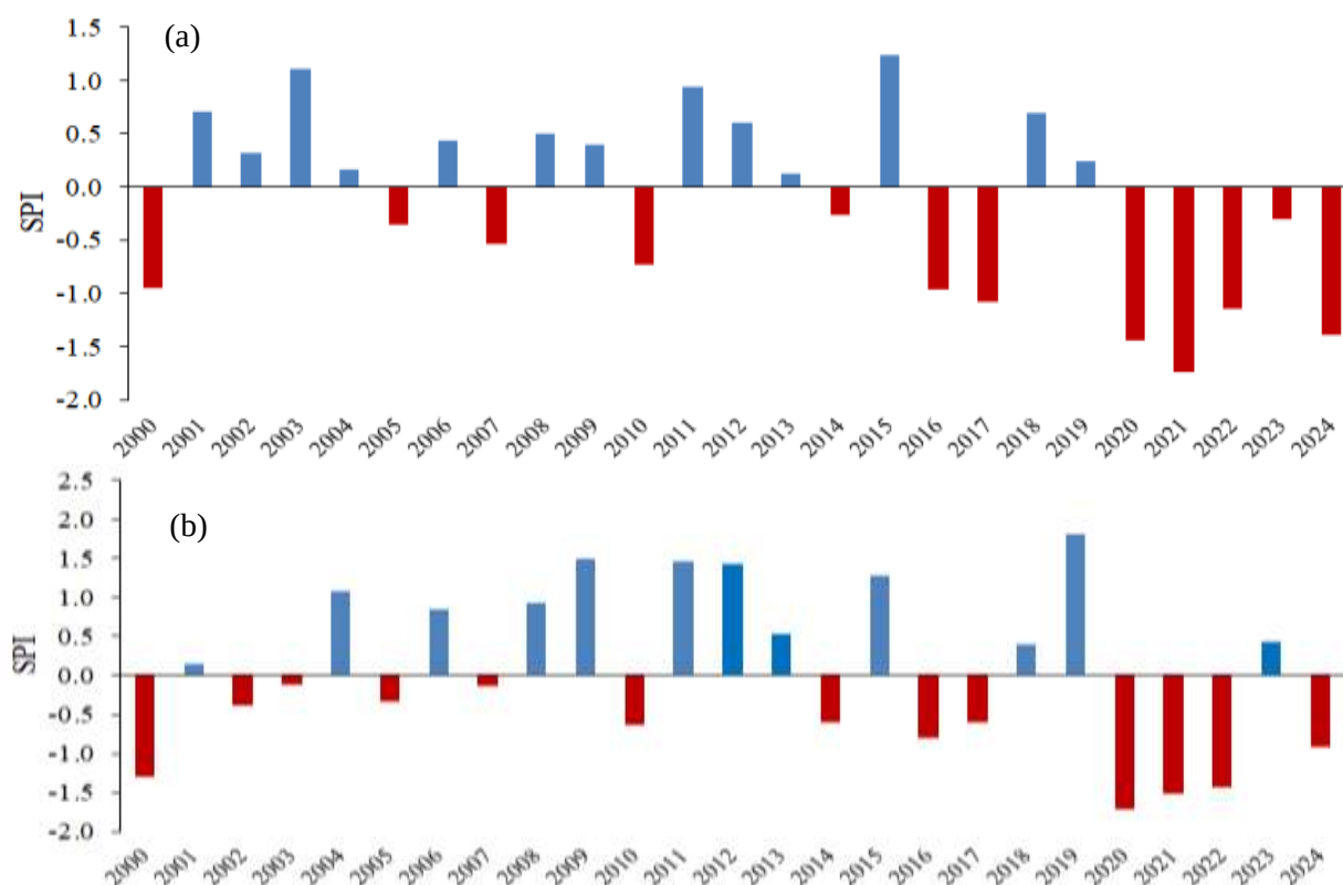
شکل ۷. مقادیر شاخص SPI سالانه (۱۲ ماهه) در ایستگاه بلغور (a) و در ایستگاه دیزباد علیا (b) طی سال‌های ۲۰۲۴-۲۰۰۰
