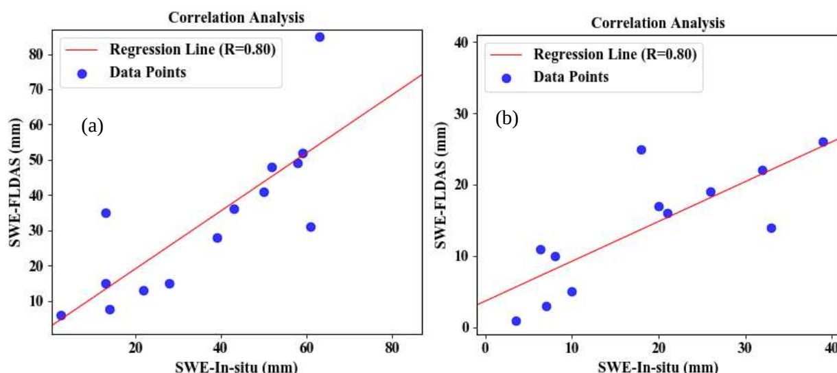
شکل ۸. نمودار همبستگی بین آب معادل برف (SWE) داده‌های ماهواره (FLDAS) و ایستگاه‌های برف‌سنجی (In-situ) در ایستگاه فریزی (a) و کریم‌آباد (b)
