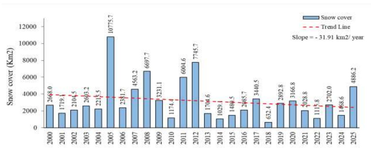
شکل ۲. نمودار تغییرات مساحت سطح پوشش برف سالانه استان خراسان رضوی در طی دوره ۲۰۲۵-۲۰۰۰
