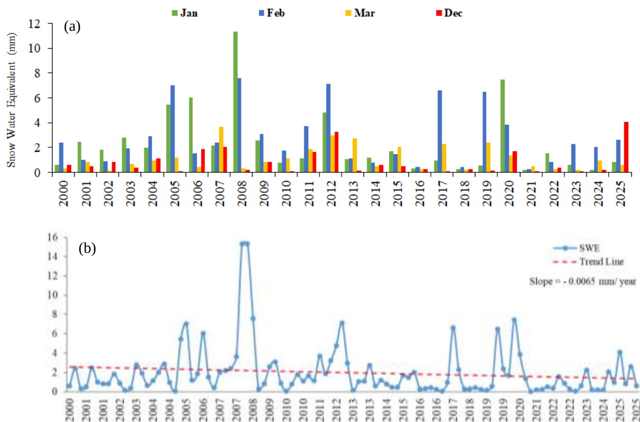
شکل ۵. نمودار میانگین ماهانه سری زمانی آب معادل برف (SWE) (a) و روند تغییرات بلند مدت آن (b) در طی دوره ۲۰۲۵-۲۰۰۰
