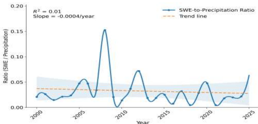
شکل ۶. نسبت آب معادل برف (SWE) به بارش سالانه (Rainfall) در طول دوره آماری ۲۰۲۵-۲۰۰۰
