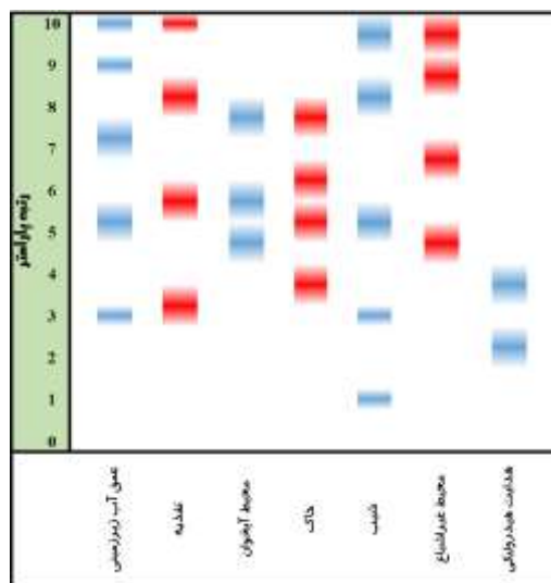
(ب) تغییرات رتبه پارامترهای شاخص DRASTIC
