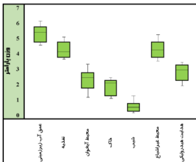
(الف) تغییرات وزن پارامترهای شاخص DRASTIC
