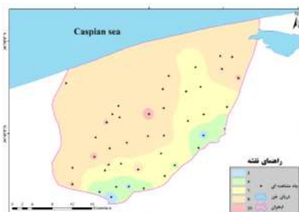
الف) رتبه‌بندی عمق آب زیرزمینی در Q75
