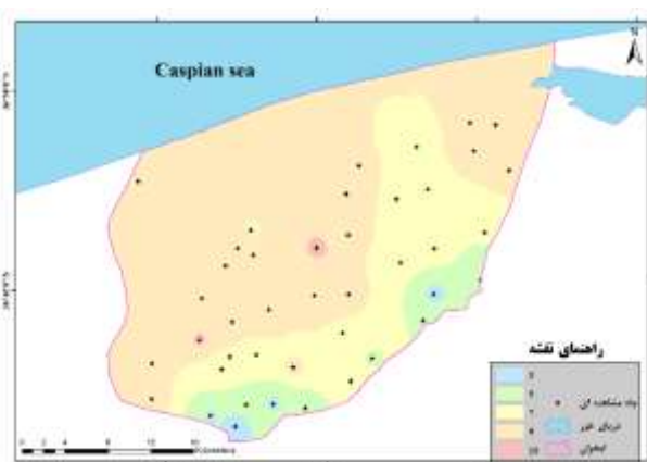
ب) رتبه‌بندی عمق آب زیرزمینی در Q50
