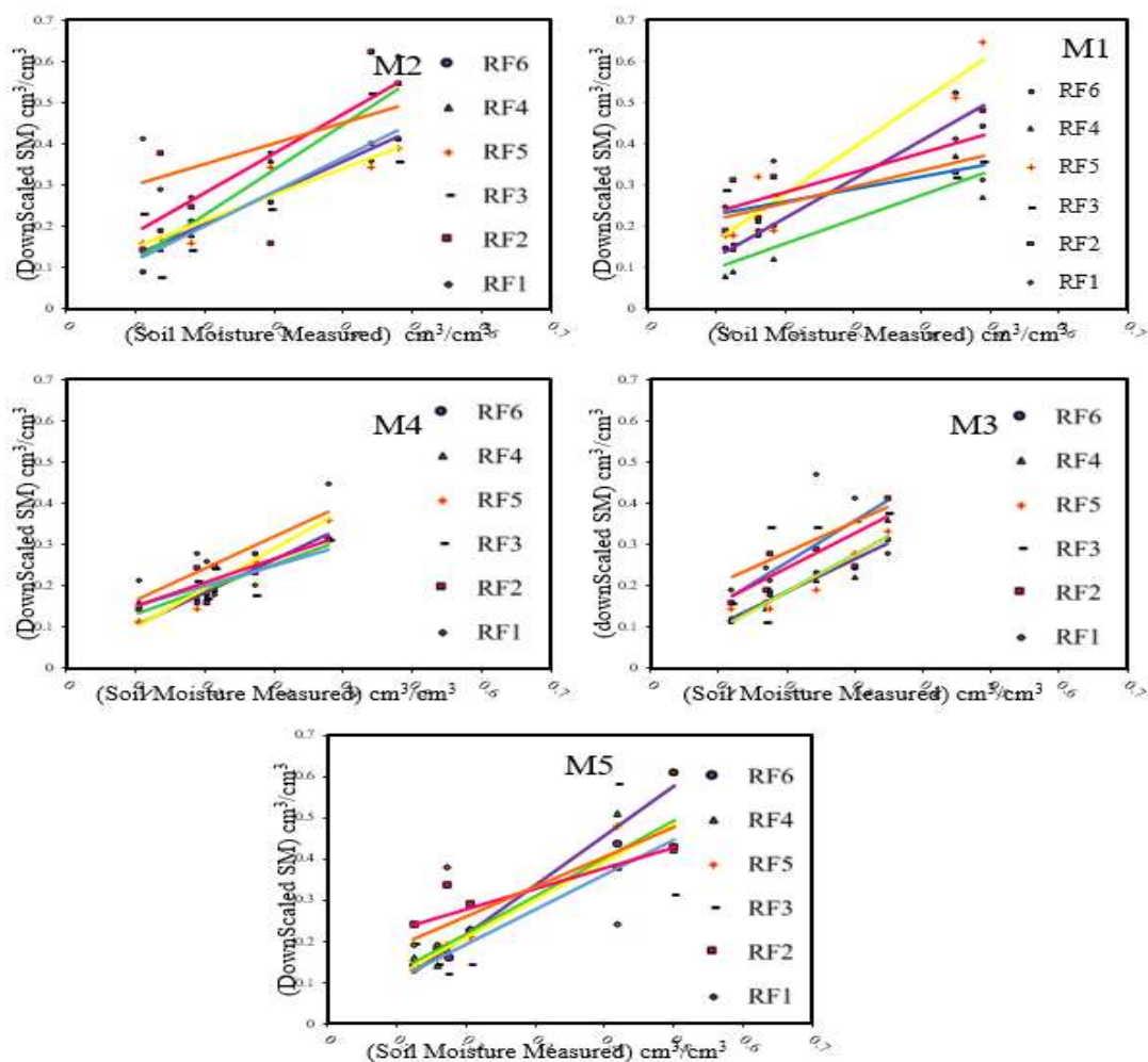
شکل ۵. نمودار پراکندگی رطوبت خاک اندازه‌گیری شده در مزرعه و ریزمقیاس‌سازی تا یک کیلومتر در سناریوهای تعریف شده
