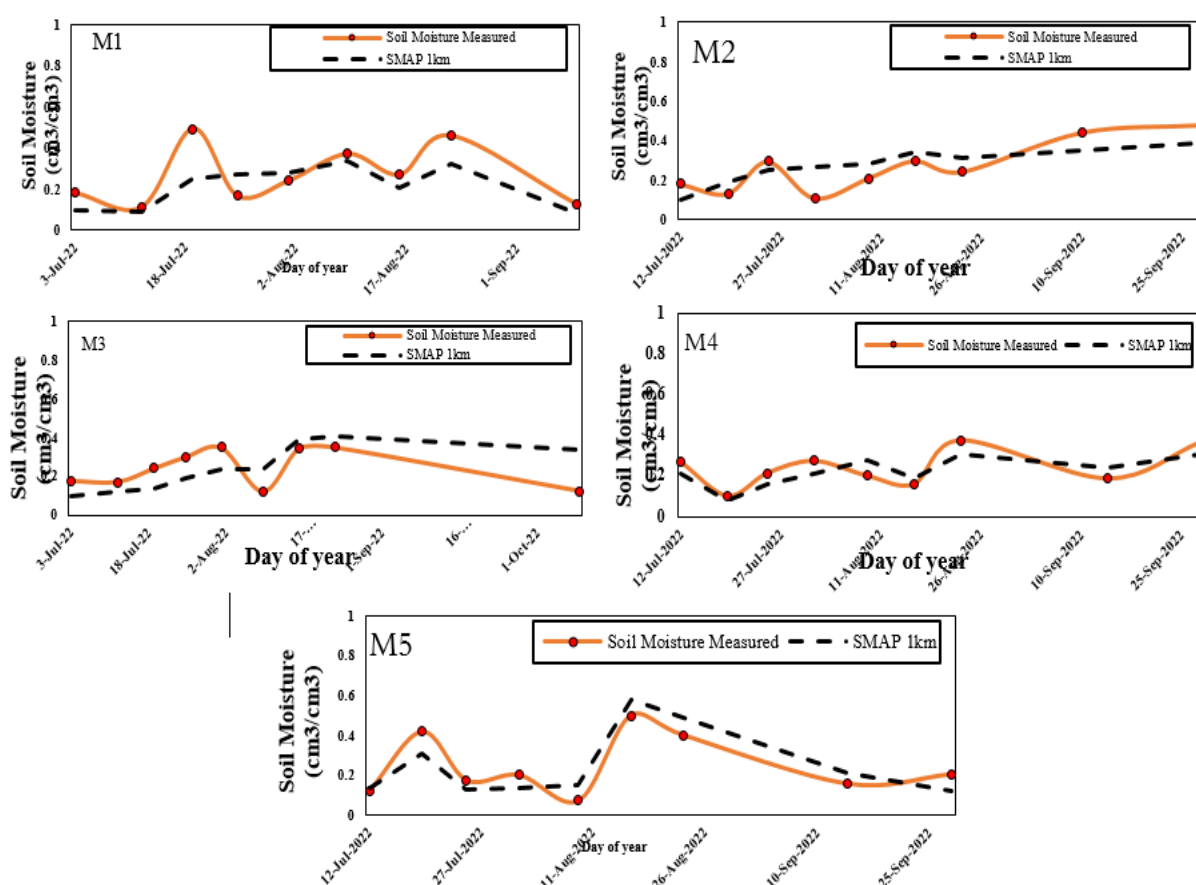
شکل ۶. نمودار سری زمانی رطوبت خاک اندازه‌گیری شده در مزارع مورد بررسی و مقایسه آن با مقادیر برآورد شده توسط SMAP 1km ریزمقیاس شده
