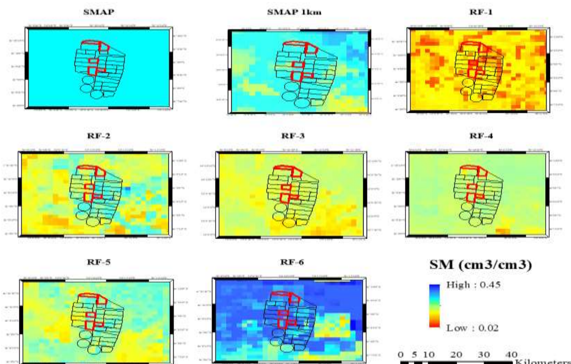
شکل ۸. بررسی پراکندگی تغییرات مکانی رطوبت خاک بر اساس سناریوهای تعریف شده و ماهواره SMAP
