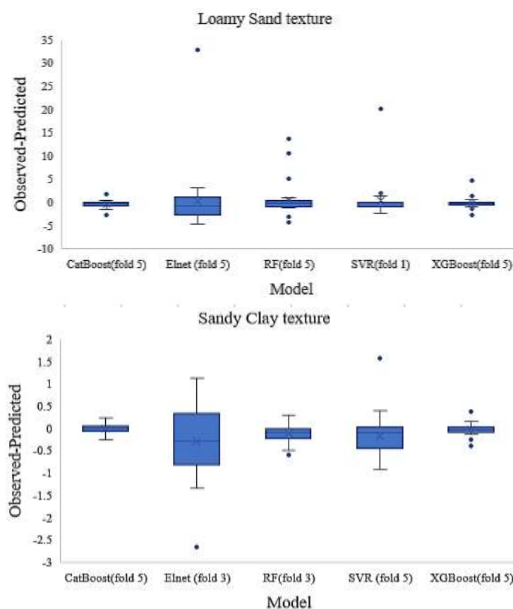
شکل ۲. نمودار جعبه‌ای خطای پیش‌بینی مدل‌های مورد بررسی در تخمین عمق نفوذ در پیاز رطوبتی
