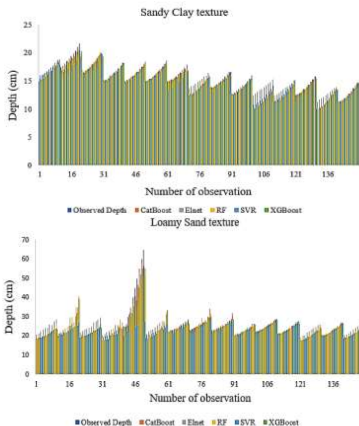
شکل ۳. مقایسه عملکرد مدل‌های مورد بررسی در پیش‌بینی عمق نفوذ پیاز رطوبتی
