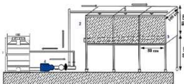
شکل ۱. نمای کلی مدل آزمایشگاهی ساخته شده شامل ۱- مخزن آب ۲- مخزن خاک ۳- لوله زهکش ۴- پمپ آب ۵- قطره چکان
