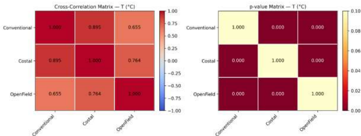
شکل ۷. ماتریس همبستگی پیرسون و سطح معنی‌داری آماری (P-VALUE) برای داده‌های دمای هوا در بین انواع محیط‌ها
