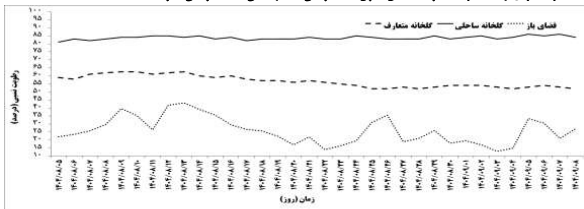
شکل ۳. نمودار تغییرات رطوبت نسبی هوا در دوره کشت محصول
