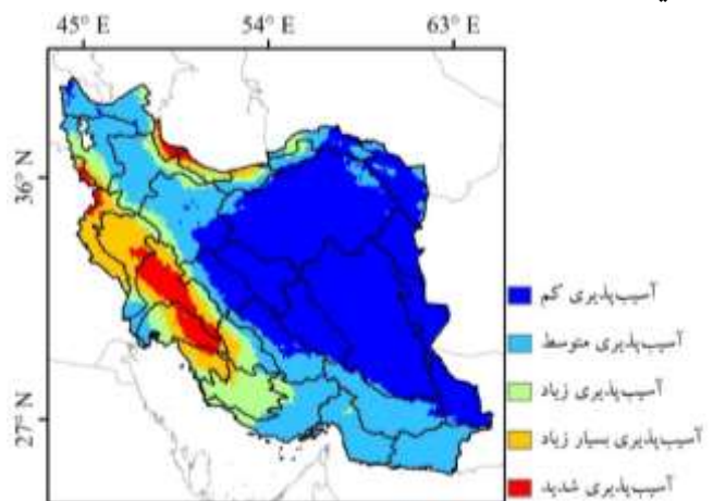
شکل ۵. مدل‌سازی فضایی آسیب‌پذیری حوضه‌های آبخیز ایران در برابر بارش‌های فرین مبتنی بر روش آنتروپی شانون. طیف رنگی نشان‌دهنده کلاس‌های آسیب‌پذیری وزنی شده از شاخص‌های شدت و فراوانی بارش فرین است.
