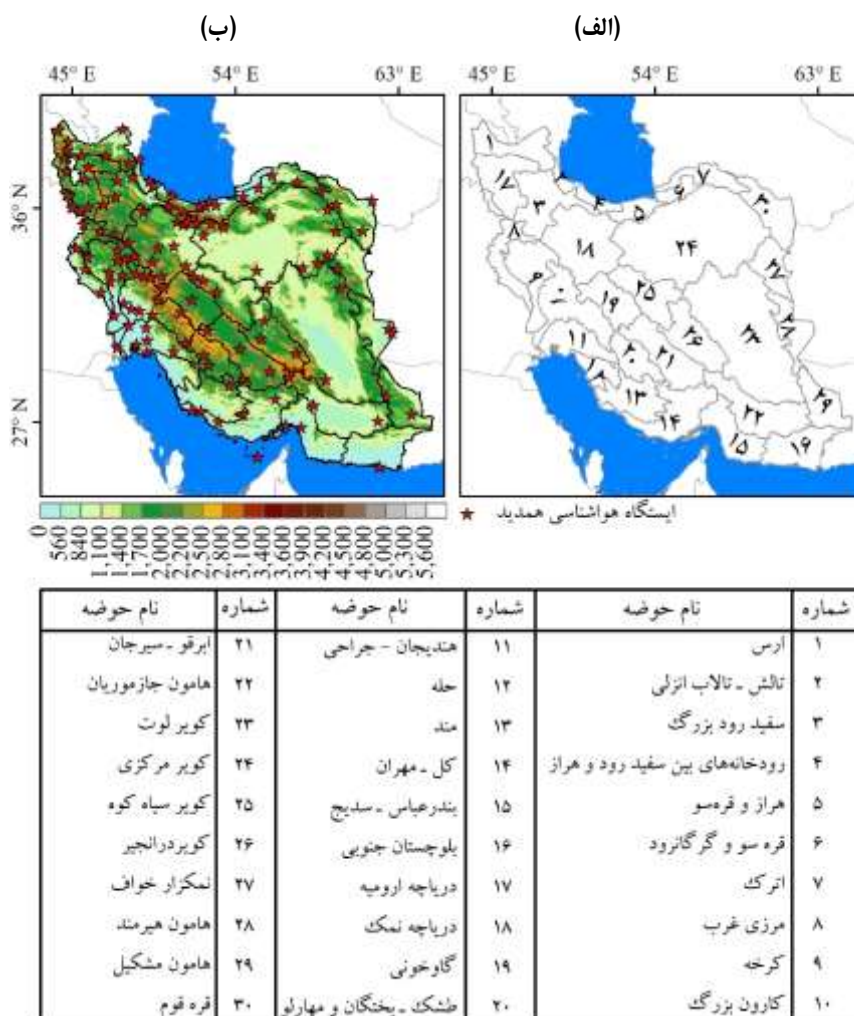
شکل ۱. موقعیت منطقه مورد مطالعه. الف) موقعیت ۳۰ حوضه آبخیز مورد بررسی در ایران و ب) مدل رقومی ارتفاعی و پراکنش ایستگاه‌های هواشناسی همدید
