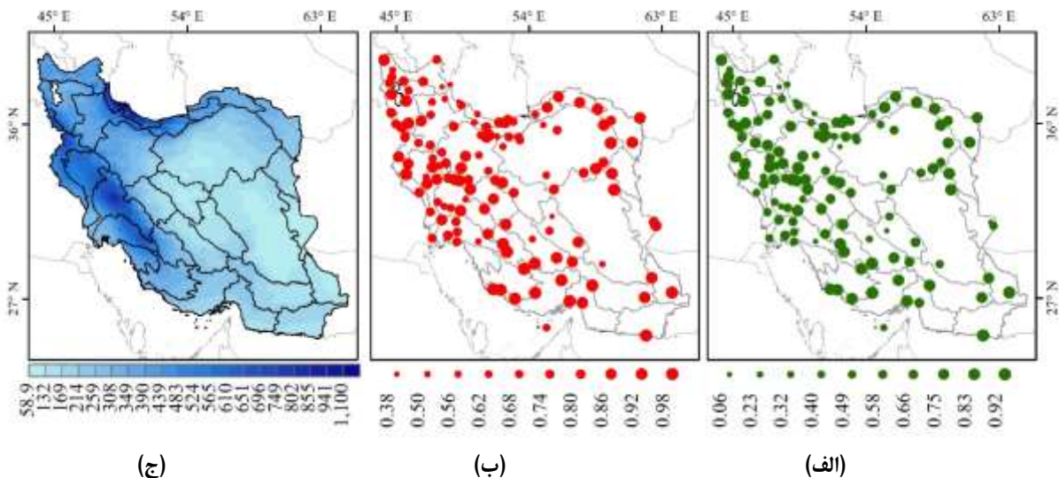
شکل ۲. توزیع مکانی میانگین بارش سالانه ایران (۲۰۲۰-۲۰۰۱) و ارزیابی فضایی کارایی محصول ماهواره‌ای GPM-IMERG. (الف) سنجه کارایی کلینگ-گوپتا (KGE) برای ۱۲۸ ایستگاه هواشناسی همدید در برابر داده‌های GPM-IMERG، (ب) شاخص‌های توافق ویلموت، (ج) میانگین سالانه بارش (واحد: میلی‌متر)
