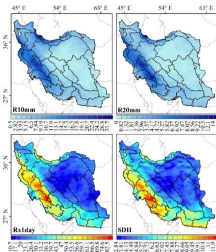
شکل ۳. توزیع مکانی بیشینه بارش یک‌روزه ( Rx1day ) (واحد: میلی‌متر)، تعداد روزهای همراه با بارش سنگین ( R10mm ) (واحد: روز)، و بسیار سنگین ( R20mm ) (واحد: روز) و شاخص شدت بارش روزانه ( SDII ) (واحد: میلی‌متر/روز) با برآوردهای ماهواره‌ای GPM-IMERG.
