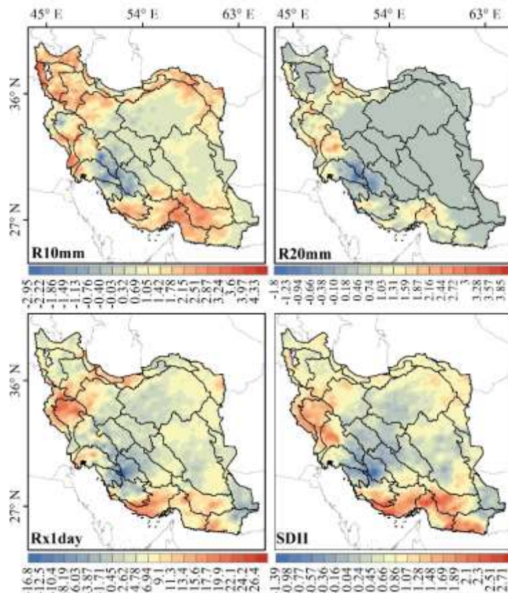
شکل ۴. روند بیشینه بارش یک‌روزه (Rx1day) (واحد: میلی‌متر/دهه)، تعداد روزهای همراه با بارش سنگین (R10mm) (واحد: روز/دهه)، و بسیار سنگین (R20mm) (واحد: روز/دهه) و شاخص شدت بارش روزانه (SDII) (واحد: میلی‌متر/روز/دهه) با برآوردهای ماهواره‌ای GPM-IMERG.
