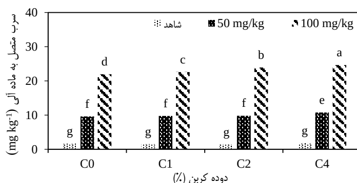
شکل ۸. مقایسه میانگین اثر متقابل سطوح مختلف دوده کربن و آلودگی خاک بر سرب متصل به ماده آلی خاک- میانگین‌های با حروف مشترک در سطح ۵ درصد آزمون توکی اختلاف معنی‌داری با هم ندارند. - (C0: شاهد، C1: یک درصد دوده کربن، C2: دو درصد دوده کربن، C4: چهار درصد دوده کربن)
