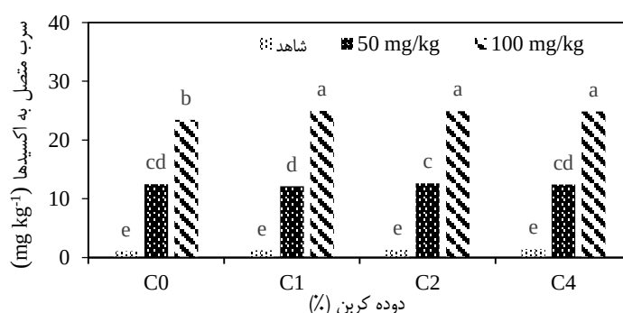
شکل ۷. مقایسه میانگین اثر متقابل سطوح مختلف دوده کربن و آلودگی خاک بر سرب متصل به اکسیدها - میانگین‌های با حروف مشترک در سطح ۵ درصد آزمون توکی اختلاف معنی‌داری با هم ندارند. - (C0: شاهد، C1: یک درصد دوده کربن، C2: دو درصد دوده کربن، C4: چهار درصد دوده کربن)
