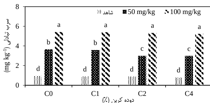
شکل ۵. مقایسه میانگین اثر متقابل سطوح مختلف دوده کربن و آلودگی خاک بر سرب تبادلی خاک- میانگین‌های با حروف مشترک در سطح ۵ درصد آزمون توکی اختلاف معنی‌داری با هم ندارند. - (C0: شاهد، C1: یک درصد دوده کربن، C2: دو درصد دوده کربن، C4: چهار درصد دوده کربن)
