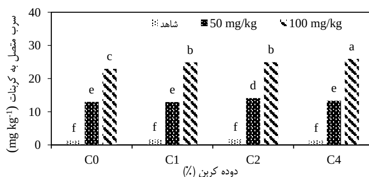
شکل ۶. مقایسه میانگین اثر متقابل سطوح مختلف دوده کربن و آلودگی خاک بر سرب کربنات‌ه خاک- میانگین‌های با حروف مشترک در سطح ۵ درصد آزمون توکی اختلاف معنی‌داری با هم ندارند. - (C0: شاهد، C1: یک درصد دوده کربن، C2: دو درصد دوده کربن، C4: چهار درصد دوده کربن)
