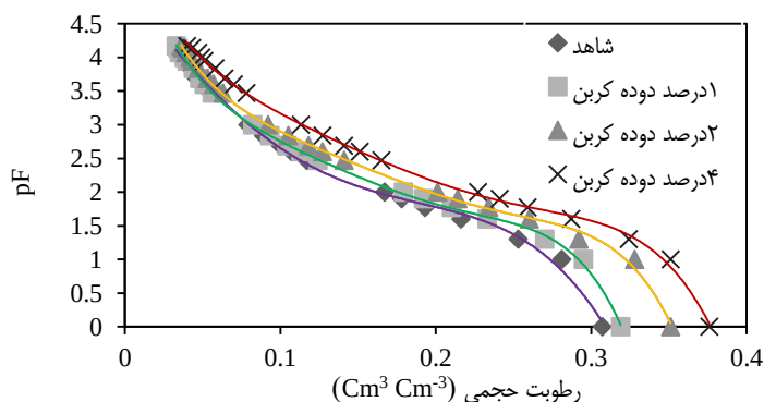
شکل ۱۲. منحنی رطوبتی خاک بر اساس معادله وانگنوختن - معلیم برای سطوح مختلف دوده کربن
