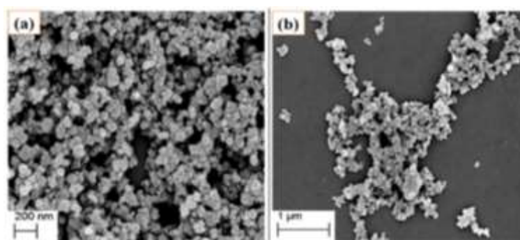
شکل ۲. تصاویر میکروسکوپ الکترونی روبشی گسیل میدانی (FESEM) دوده کربن N-330 (Paul et al., 2023)
