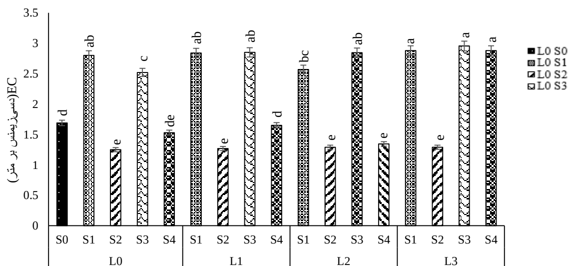
شکل ۲: مقایسه میانگین EC خاک پوششی در تیمارهای آزمایش
