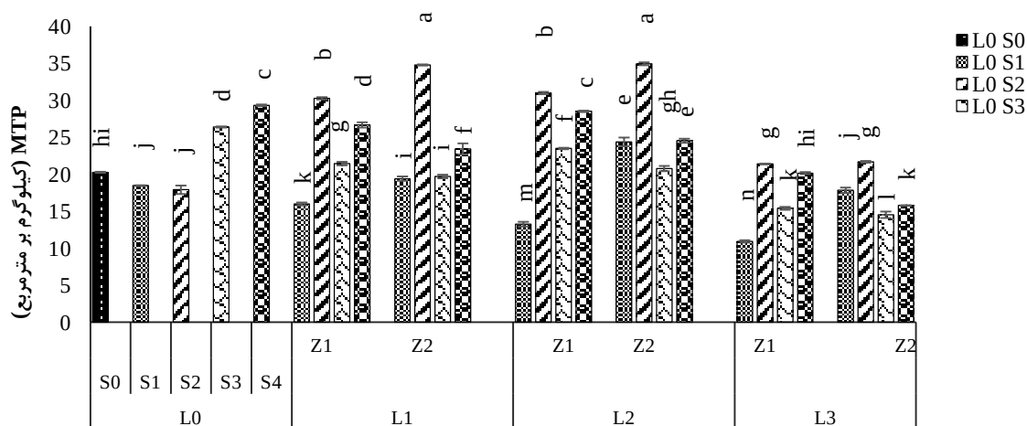
شکل ۴: مقایسه میانگین عملکرد قارچ دکمه‌ای در تیمارهای آزمایش S: نوع خاک، L: مقدار بیوجار، Z: اندازه ذرات بیوجار.
