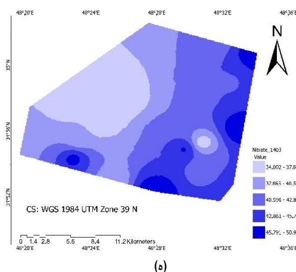
شکل ۲ - پهنه‌بندی غلظت نیترات آب زیرزمینی دشت همدان - بهار از سال ۱۳۹۹ تا ۱۴۰۳
