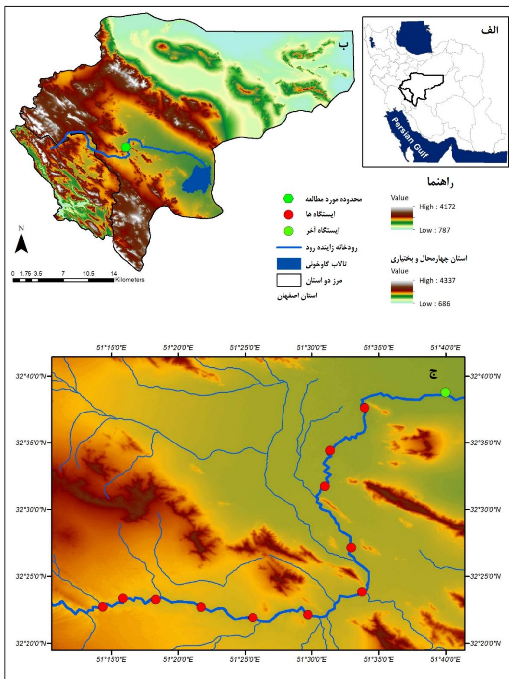
شکل ۱. موقعیت رودخانه زاینده‌رود: (الف) مرزهای دو استان، (ب) کل مسیر ۳۵۰ کیلومتری رودخانه از مبدأ (استان چهارمحال و بختیاری) تا مقصد (تالاب گاوخونی)، (ج) موقعیت ۱۲ مقطع عرضی در بازه انتخابی ۹۱ کیلومتری (منطقه مورد مطالعه).
