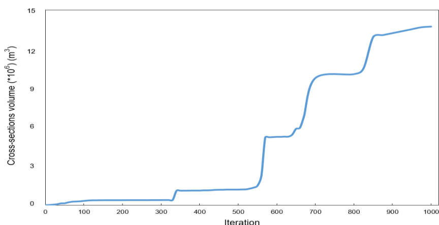
شکل ۸. روند بهینه‌سازی حجم لایروبی با استفاده از الگوریتم SBOA طی ۱۰۰۰ تکرار.
