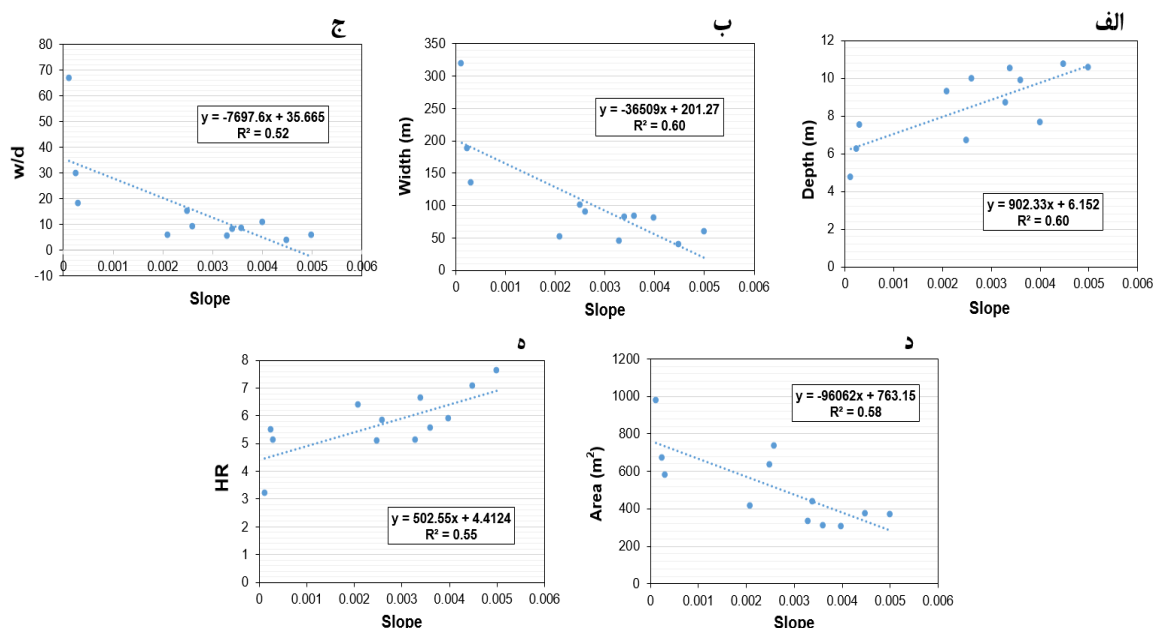
شکل ۶. فرآیند تغییرات بین عمق (الف)، عرض (ب)، عرض به عمق (ج)، مساحت (د) و شعاع هیدرولیکی (HR) (ه) با شیب طولی رودخانه.
