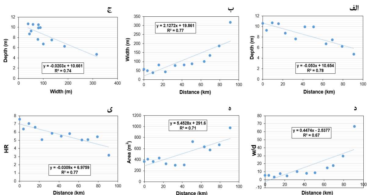
شکل ۵. فرآیند تغییرات بین عمق و فاصله (الف)، عرض و فاصله (ب)، تغییرات بین عرض و عمق (ج)، عرض به عمق و فاصله (د)، تغییرات بین مساحت و فاصله (ه) و شعاع هیدرولیکی (HR) و فاصله (و).
