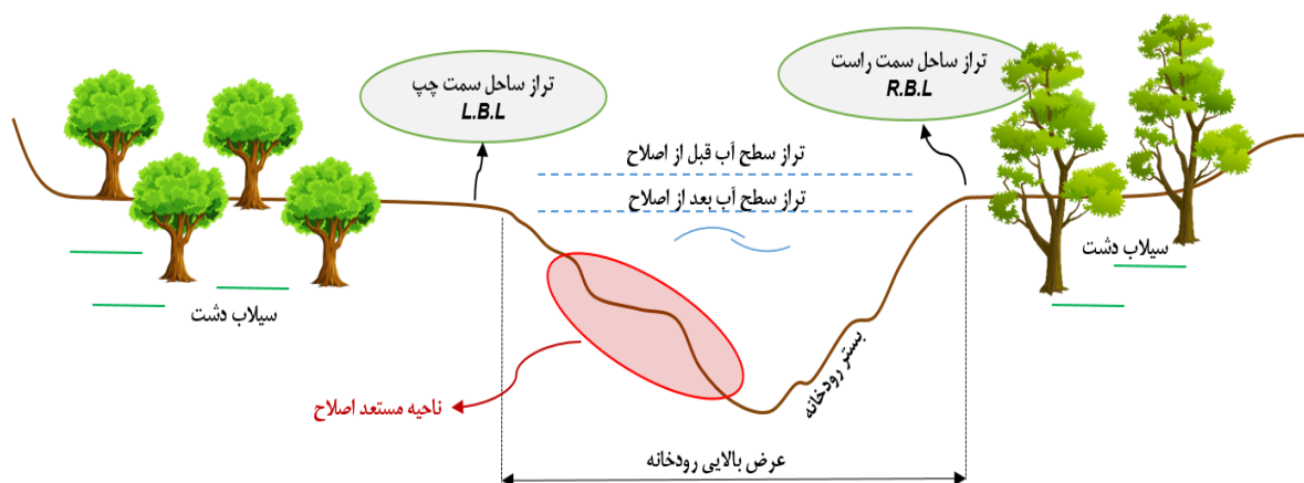
شکل ۳. پارامترهای رودخانه در داخل و خارج از کانال شامل: سیلاب‌دشت‌ها، سطح آب، عرض رودخانه و سطوح کرانه‌های راست و چپ.
