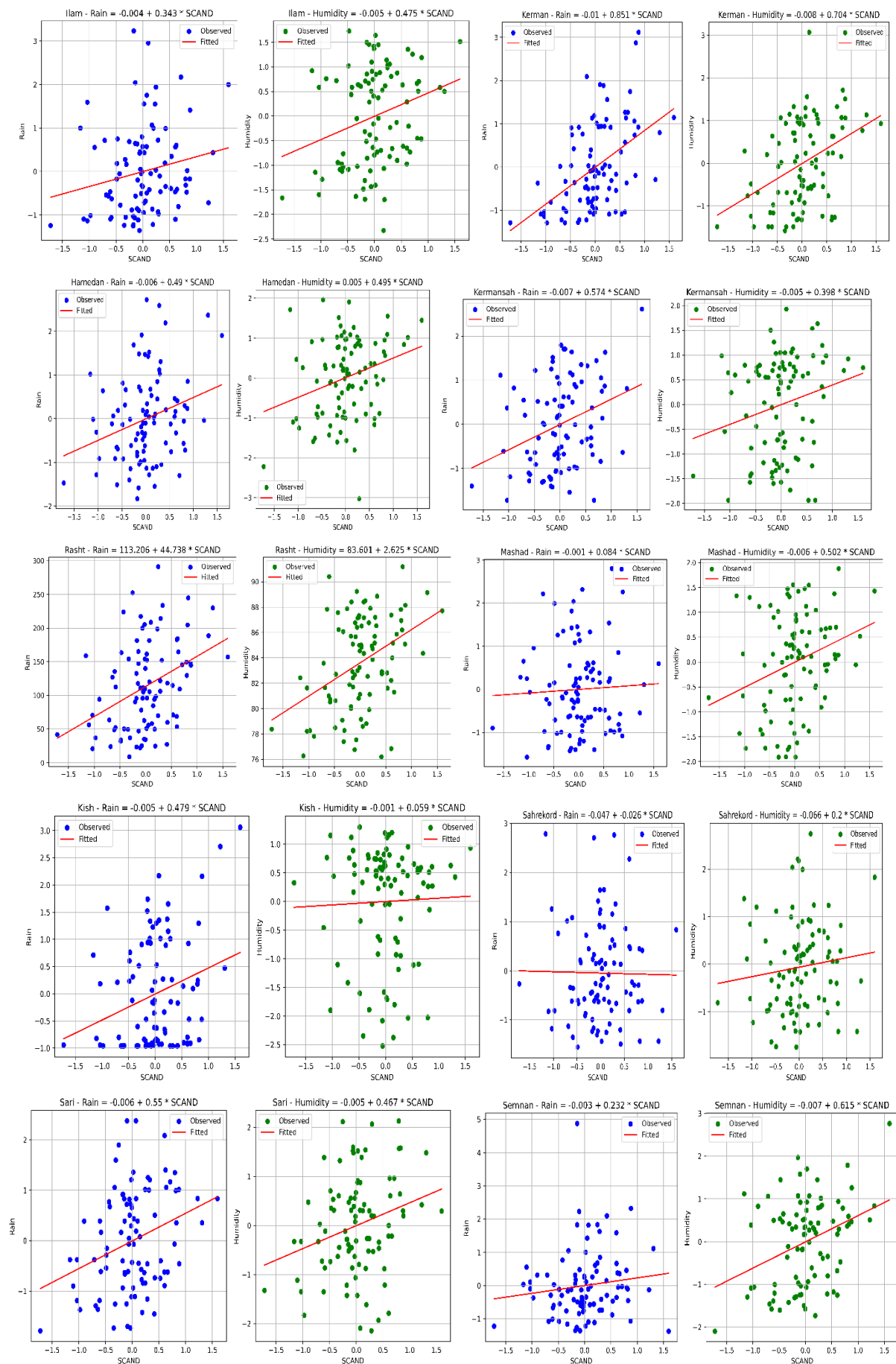
ادامه شکل ۹: نمودار رگرسیون مولفه‌های هواشناسی با شاخص اسکاندیناوی پس از آنالیز p.c.a
