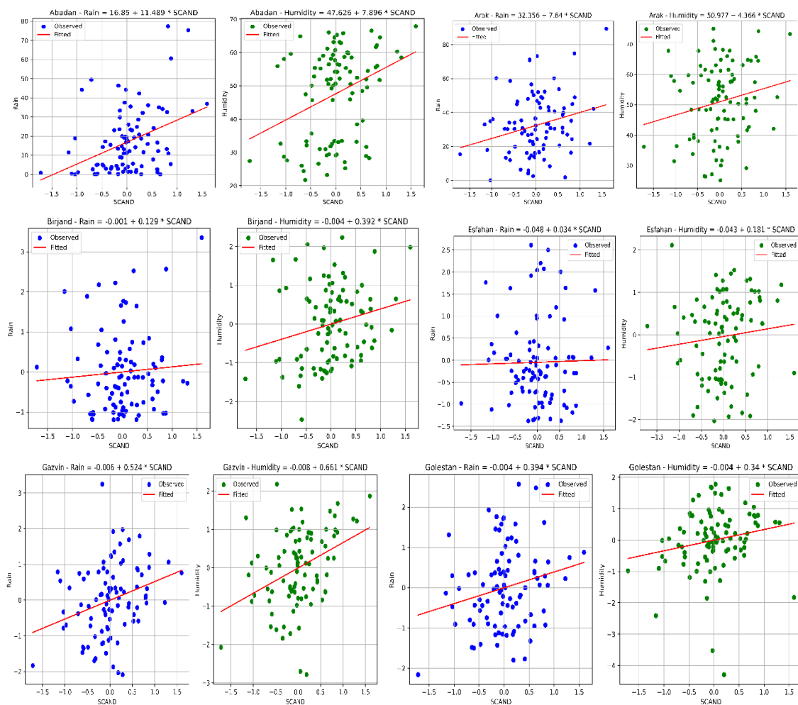
شکل ۹: نمودار رگرسیون مولفه‌های هواشناسی با شاخص اسکاندیناوی پس از آنالیز p.c.a
