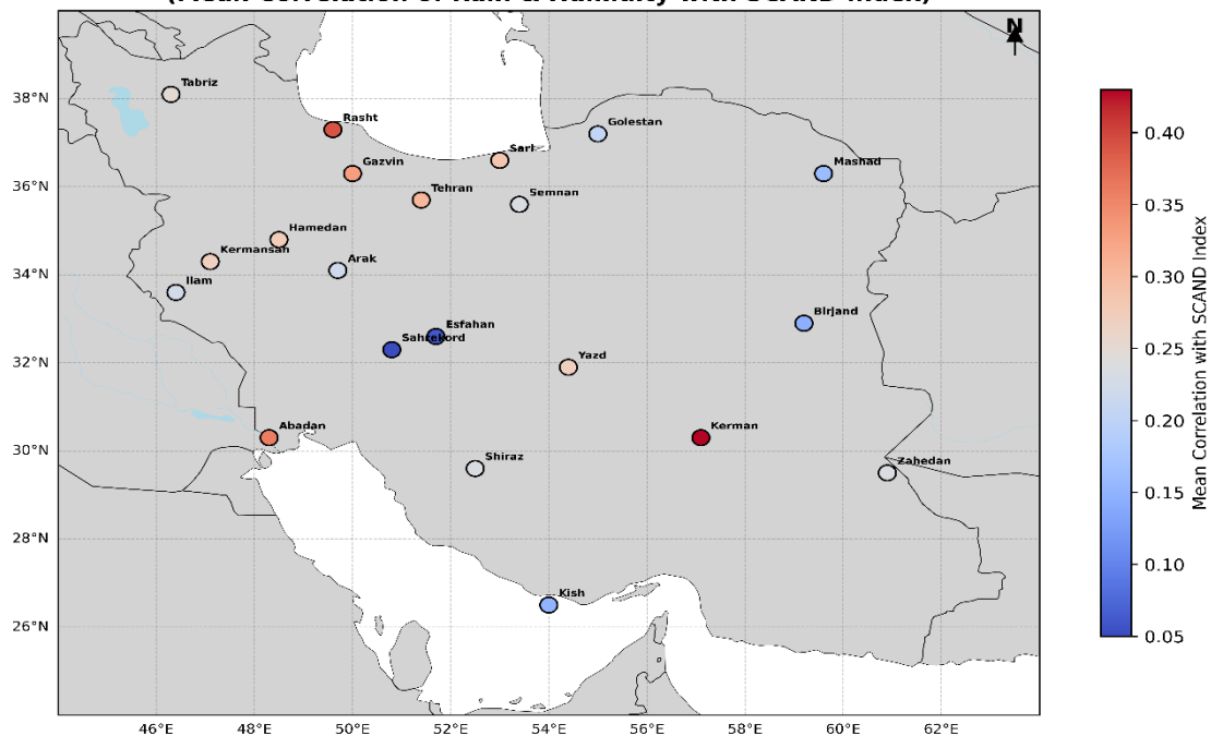
شکل ۸: میانگین همبستگی شاخص اسکاندیناوی با ایستگاه.
