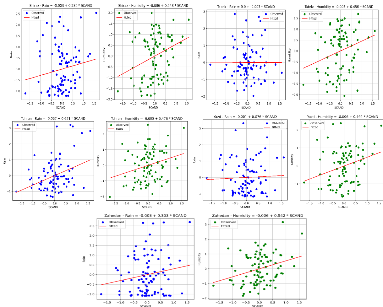
ادامه شکل ۹: نمودار رگرسیون مولفه‌های هواشناسی با شاخص اسکاندیناوی پس از آنالیز p.c.a
