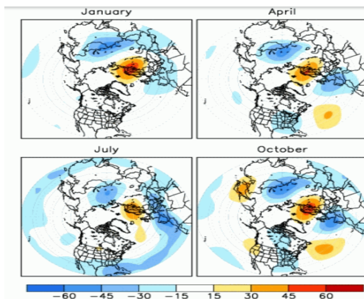
شکل ۲: الگوی فاز مثبت شاخص اسکاند در فصول مختلف در تراز ۵۰۰ هکتو پاسکال (NOAA)
