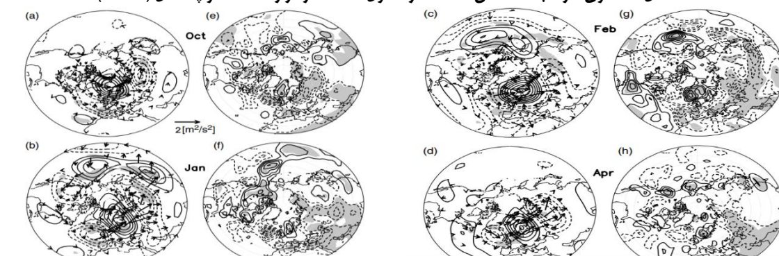
شکل ۳: جزء افقی ۳۰۰ مگابایت شار فعالیت موج (فلش) مرتبط با الگوی SCA برای (a) اکتبر، (b) ژانویه،
