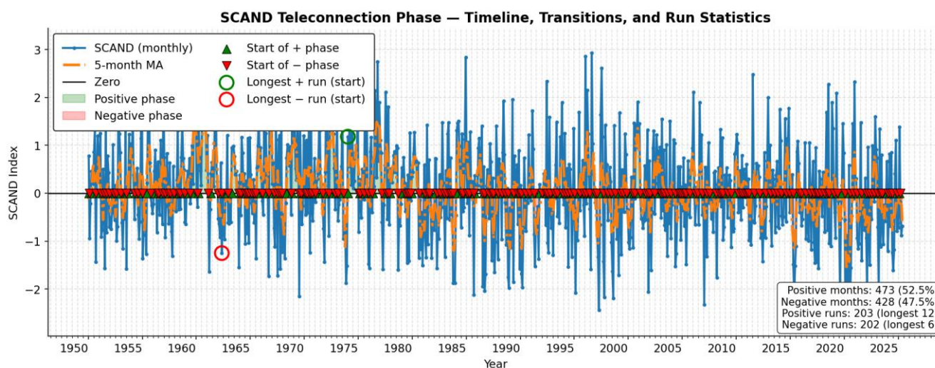
شکل ۵: نمودار شاخص منطقه اسکاندیناوی در بازه زمانی ۷۵ سال اخیر ۱۹۵۰-۲۰۲۵ (NOAA).
