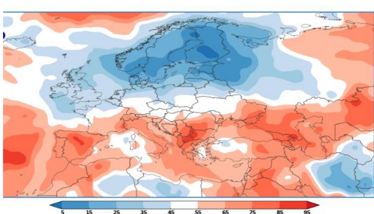
شکل ۴ ب: آنومالی بارش میانگین سه ماهه زمستان اروپا و خاورمیانه و ایران (ژانویه، فوریه و مارچ) بازه زمانی ۱۹۹۰-۲۰۲۰ (واحد میلی متر) (World Climate Service))
