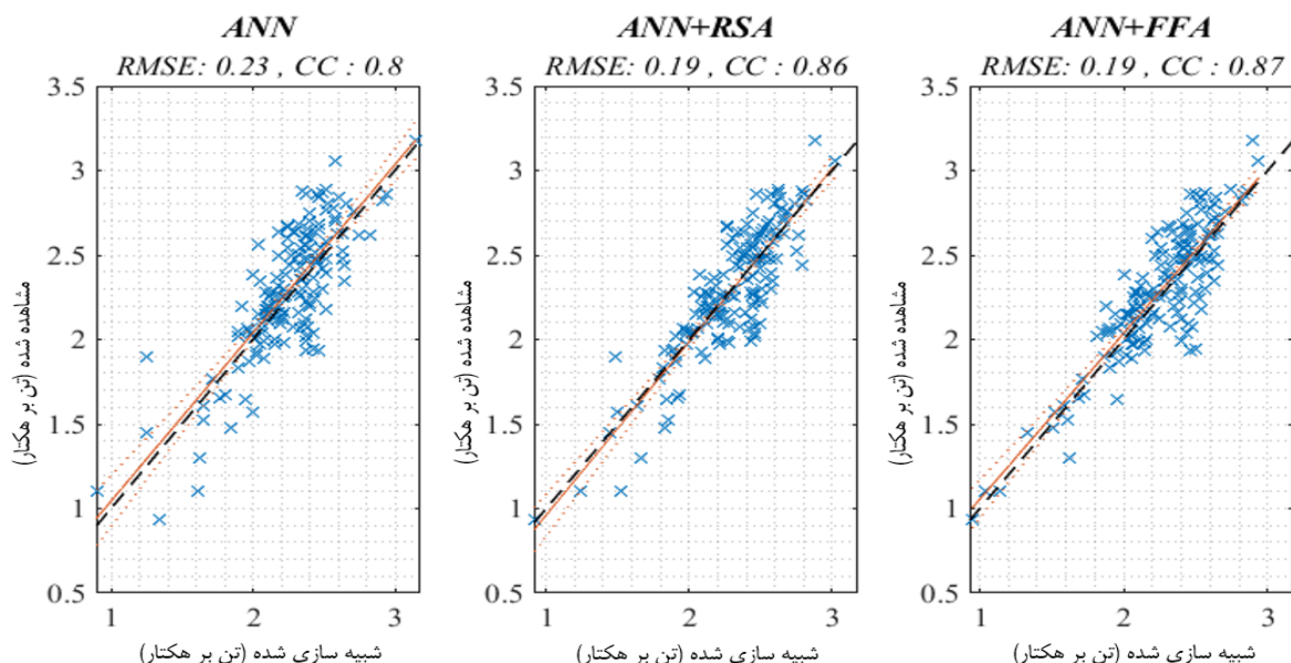
شکل ۶. مقادیر همبستگی داده‌های مشاهداتی و شبیه‌سازی شده با مدل‌های یادگیری ماشین - مرحله آزمون، (ضریب همبستگی: CC)
