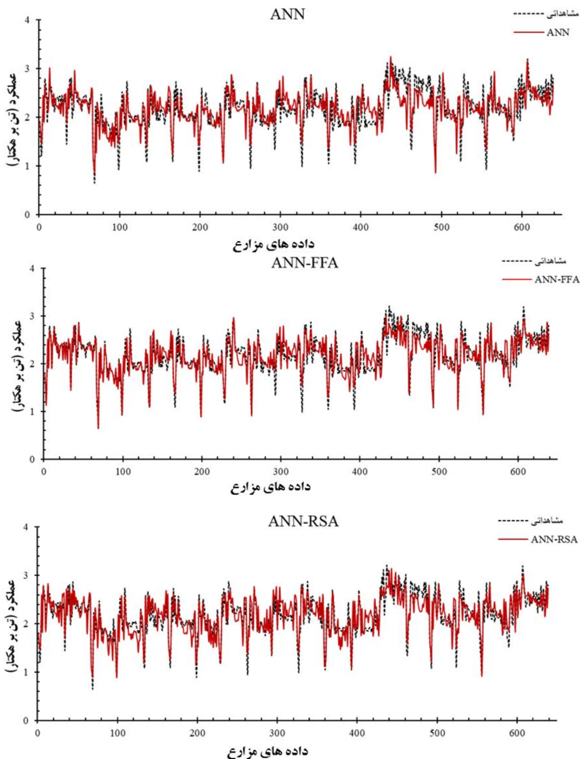
شکل ۸. نمودار سری زمانی داده‌های مشاهداتی و شبیه‌سازی شده
