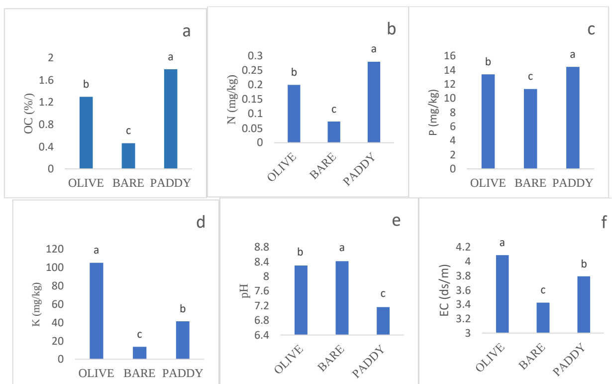
شکل ۴. مقایسه میانگین ویژگی‌های شیمیایی خاک در کاربری‌های مختلف
