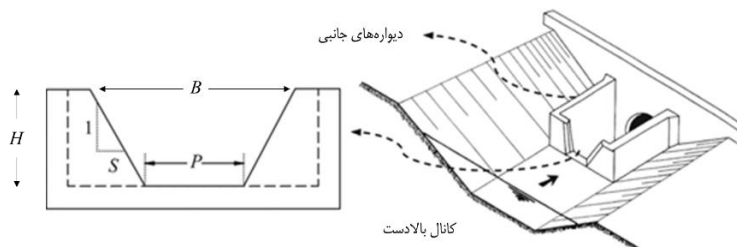
شکل ۱. شکاف کنترل دوزنقه‌ای (Vatankhah, 2013a)
