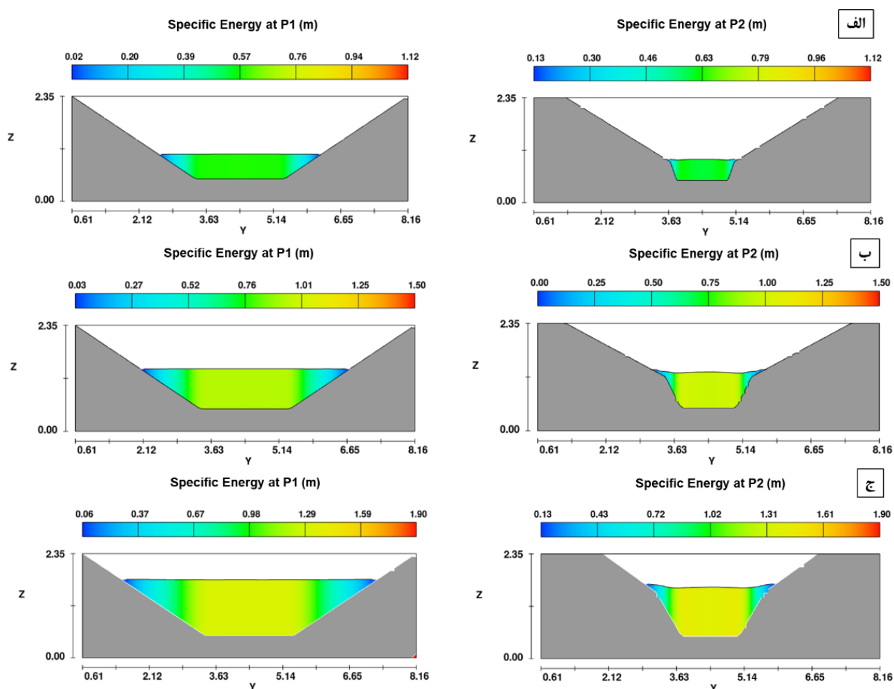
شکل ۱۰. مقایسه گرافیکی انرژی مخصوص جریان در نقاط P1 و P2 برای حالت‌های هیدرولیکی الف (۱)، ب (۲) و ج (۳)
