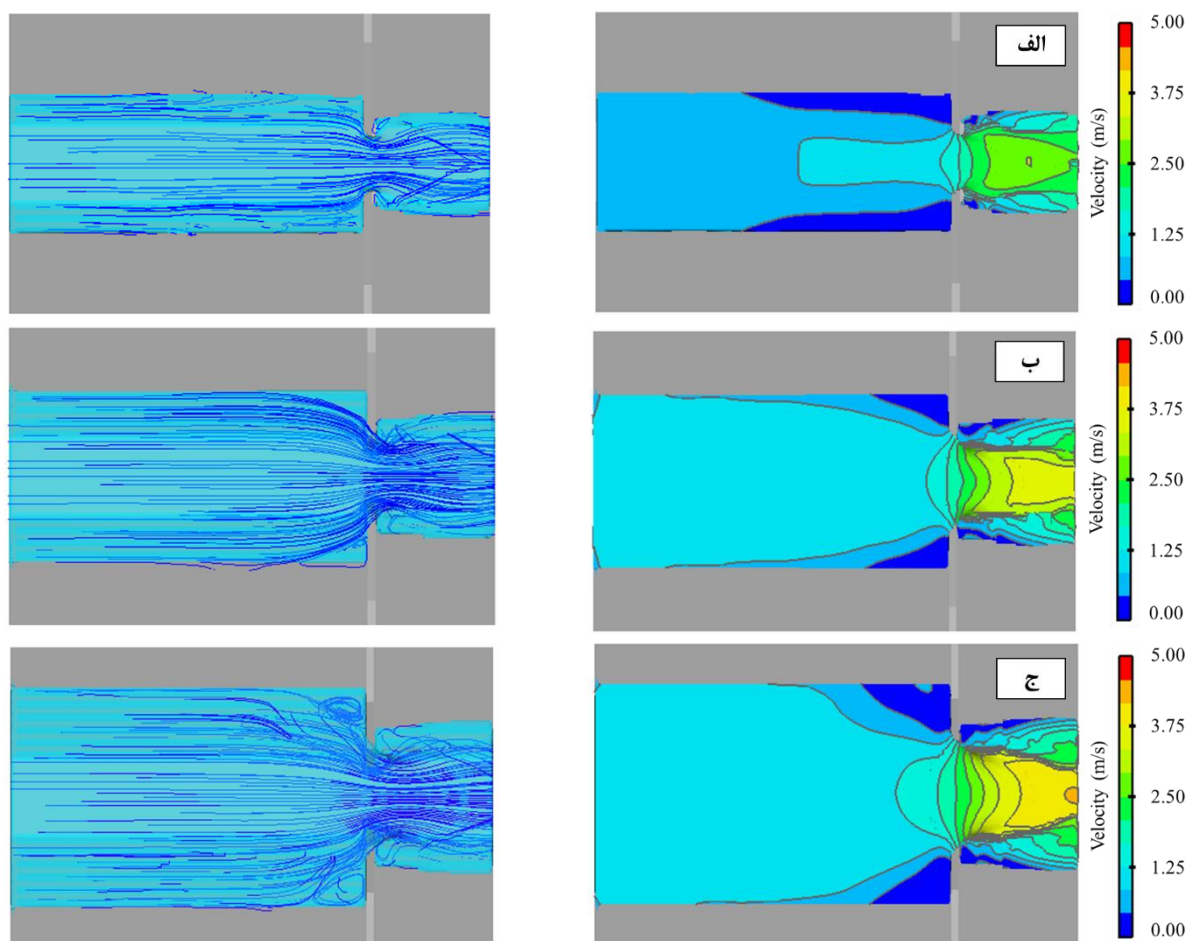
شکل ۱۱. میدان توزیع سرعت و خطوط جریان در دامنه محاسباتی شبیه‌سازی به‌ازای دبی‌های الف) ۱، ب) ۲/۵ و ج) ۵ متر مکعب بر ثانیه
