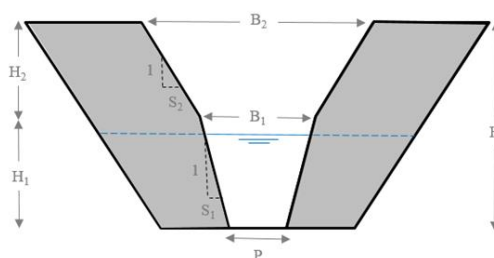
شکل ۲. شکاف کنترل مرکب دوزنقه‌ای
