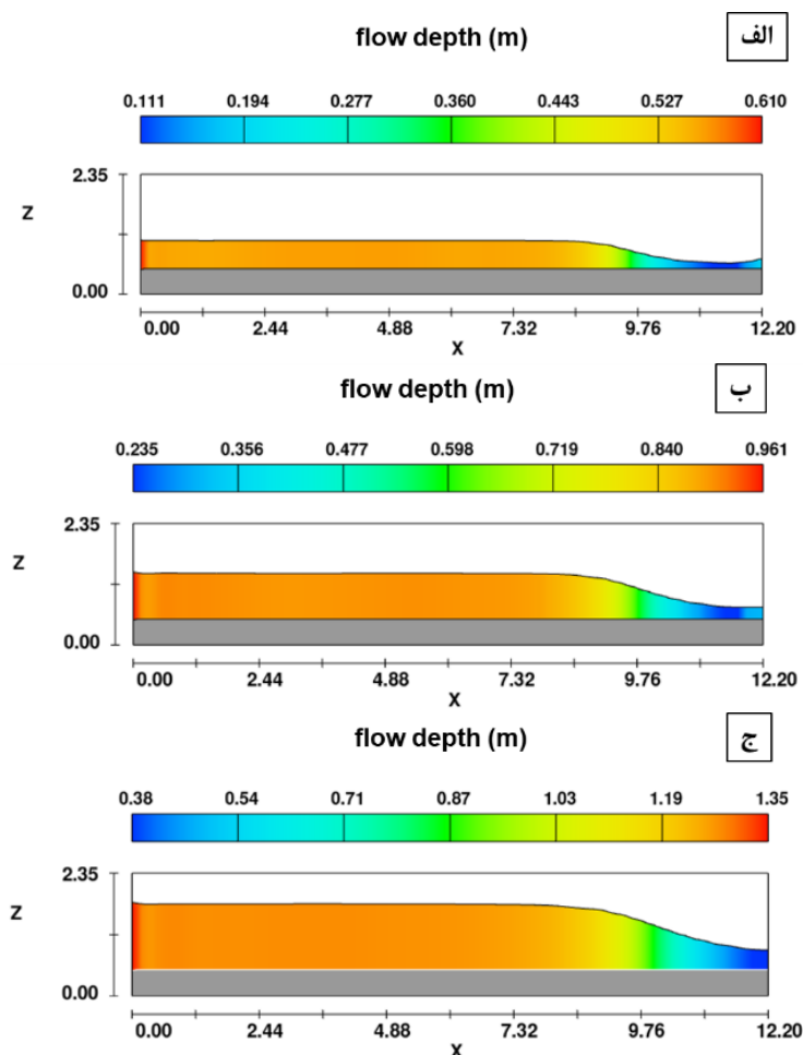
شکل ۹. نیمرخ سطح آب در حضور شکاف کنترل مرکب دوزنقه‌ای برای حالت‌های الف (۱، ب) ۲ و ج) ۳
