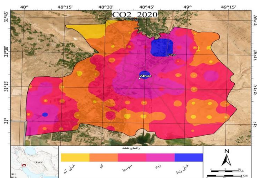
شکل ۵. تغییرات کربن دی اکسید در سال ۲۰۲۰
