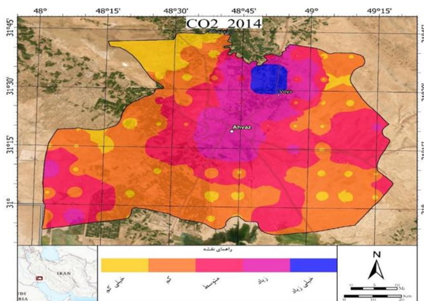
شکل ۴. تغییرات انتشار \text{CO}_2 در سال ۲۰۱۴
