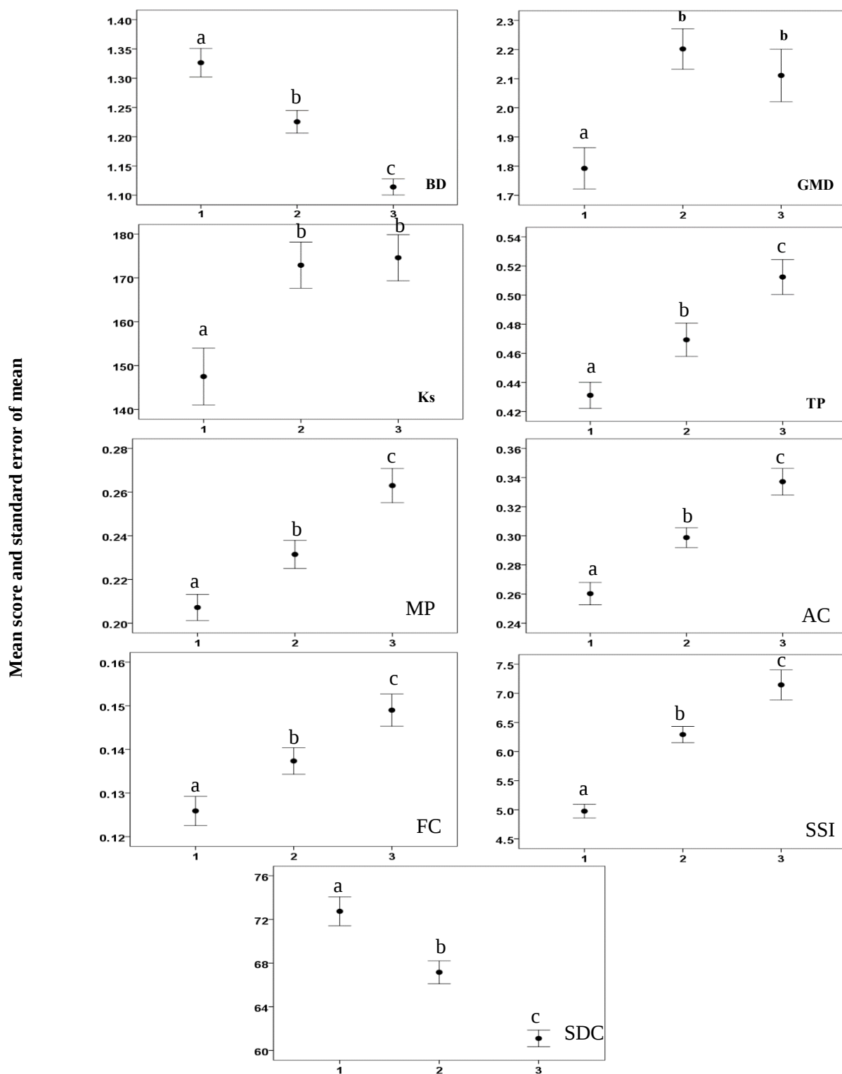
شکل ۲ - مقایسه میانگین ویژگی‌های فیزیکی خاک بین مدیریت‌های مختلف ۱- مرتع با شرایط طبیعی، ۲- مراتع با عملیات قرق و بذرپاشی ۳- مراتع نهال کاری شده. حروف انگلیسی متفاوت در هر نمودار نشان دهنده تفاوت معنی‌دار بر اساس آزمون LSD در سطح احتمال ۰/۰۵ می‌باشد. BD: Bulk density; GMD: Geometric mean diameter; Ks: Saturate hydraulic conductivity; TP: Total porosity; MP: Macro porosity; AC: Air capacity; FC: Field capacity; SSI: Soil structural index; SDC: Soil degree of compactness.
