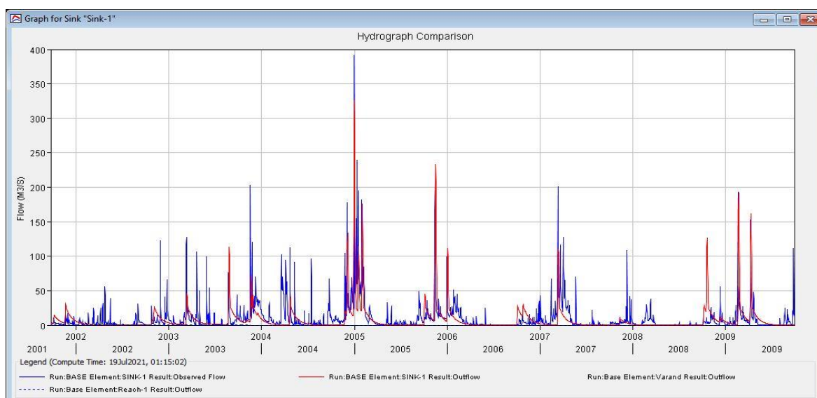
شکل ۸. هیدروگراف جریان روزانه مشاهده‌شده و شبیه‌سازی شده (۱۳۸۱-۱۳۸۸)
