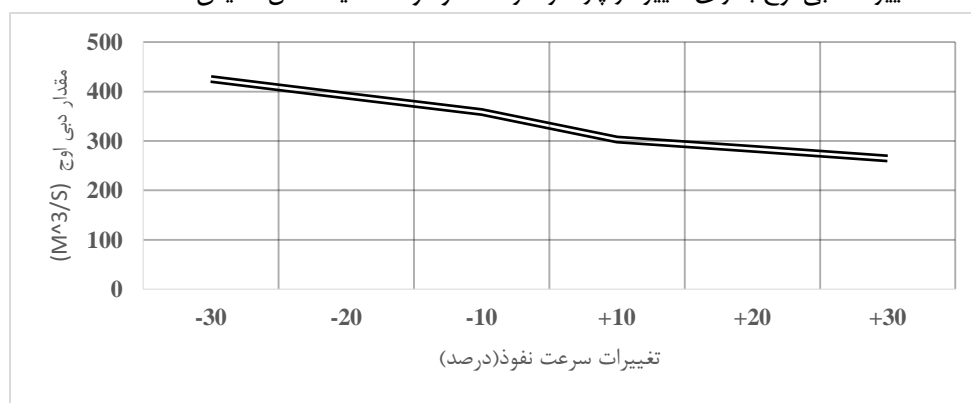
شکل ۱۰. نمودار تغییرات دبی اوج نسبت به ازای تغییرات همزمان در پارامترها
