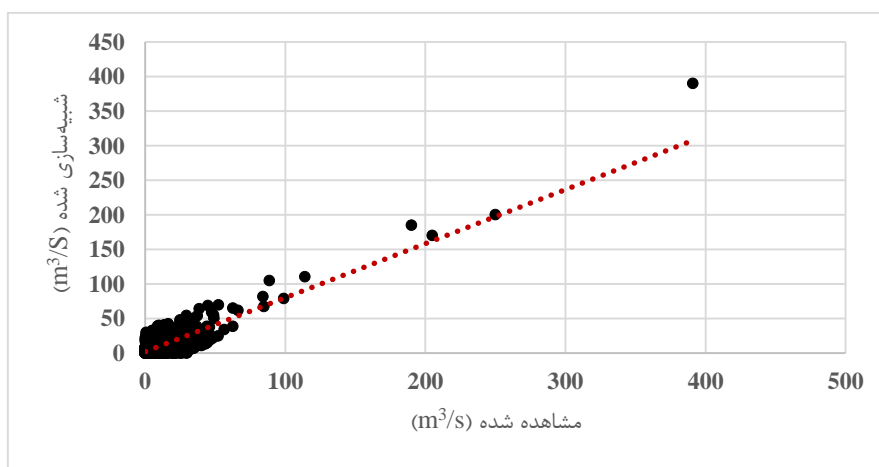
شکل ۱۲. نمودار مقایسه مقادیر دبی متوسط روزانه مشاهده شده و شبیه‌سازی شده در مرحله واسنجی (۱۳۸۱-۸۸)
