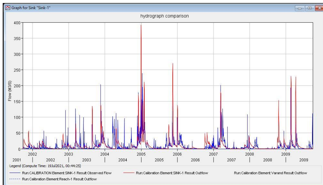
شکل ۱۱. هیدروگراف جریان روزانه مشاهده‌ای و محاسبه شده در مرحله واسنجی (۱۳۸۱-۸۸)
