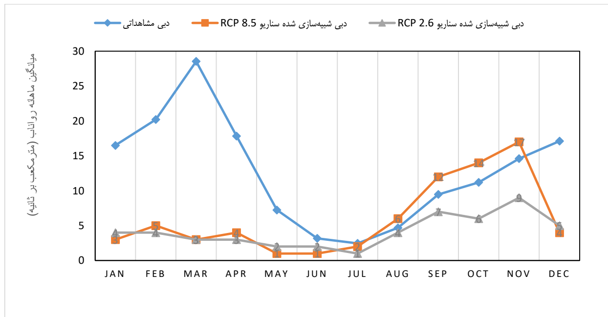
شکل ۱۵. تغییرات دبی شبیه‌سازی شده در دوره‌ی آبی نسبت به دوره‌ی پایه مشاهداتی تحت سناریوهای RCP 2.6 و RCP 8.5
