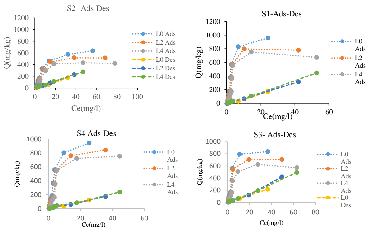
شکل ۲. نمودار جذب و واجذب بور بر روی خاک‌های مورد مطالعه، L0: نمونه شاهد (بدون لئوناردیت)، L2: کاربرد ۲ درصد لئوناردیت، L4: کاربرد ۴ درصد لئوناردیت، Ads: جذب بور، Des: واجذب بور
