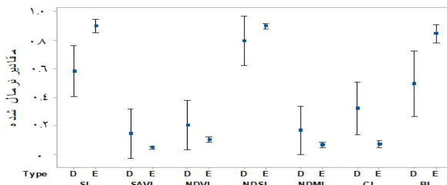
شکل ۳- نمودار تغییرات مقادیر شاخص‌های نرمال شده سنجش از دور برای سطوح فرسایشی و رسوبی
