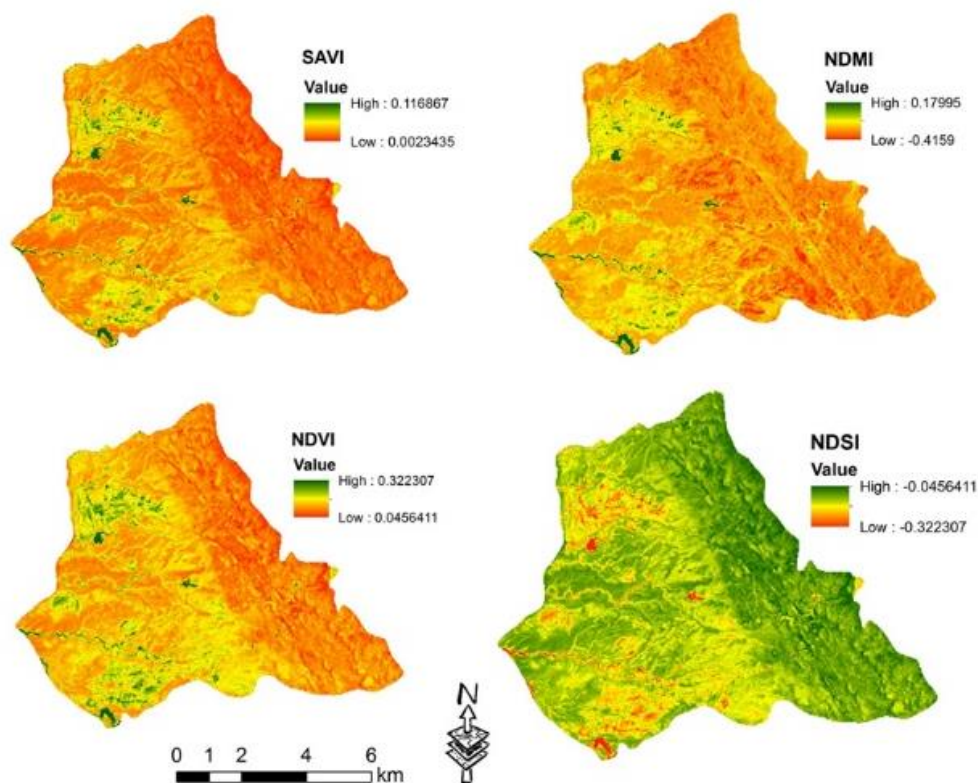
شکل ۴- نقشه‌ی توزیع مکانی شاخص‌های NDVI و NDSI، SAVI، SI، BI، CI، NDMI در منطقه‌ی مطالعاتی
