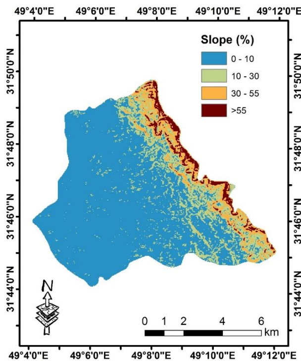
شکل ۲- نقشه‌ی پراکنش مکانی درجه شیب (%) در منطقه‌ی مطالعاتی
