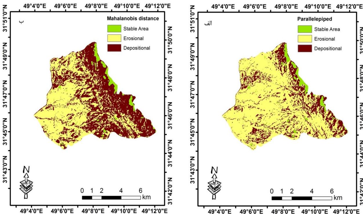
شکل ۷ - نقشه‌ی تفکیک سطوح فرسایشی و رسوبی با استفاده از الگوریتم‌های سطوح موازی (الف) و فاصله ماھالانوبی (ب) در تلفیق با شاخص‌های سنجش از دور
