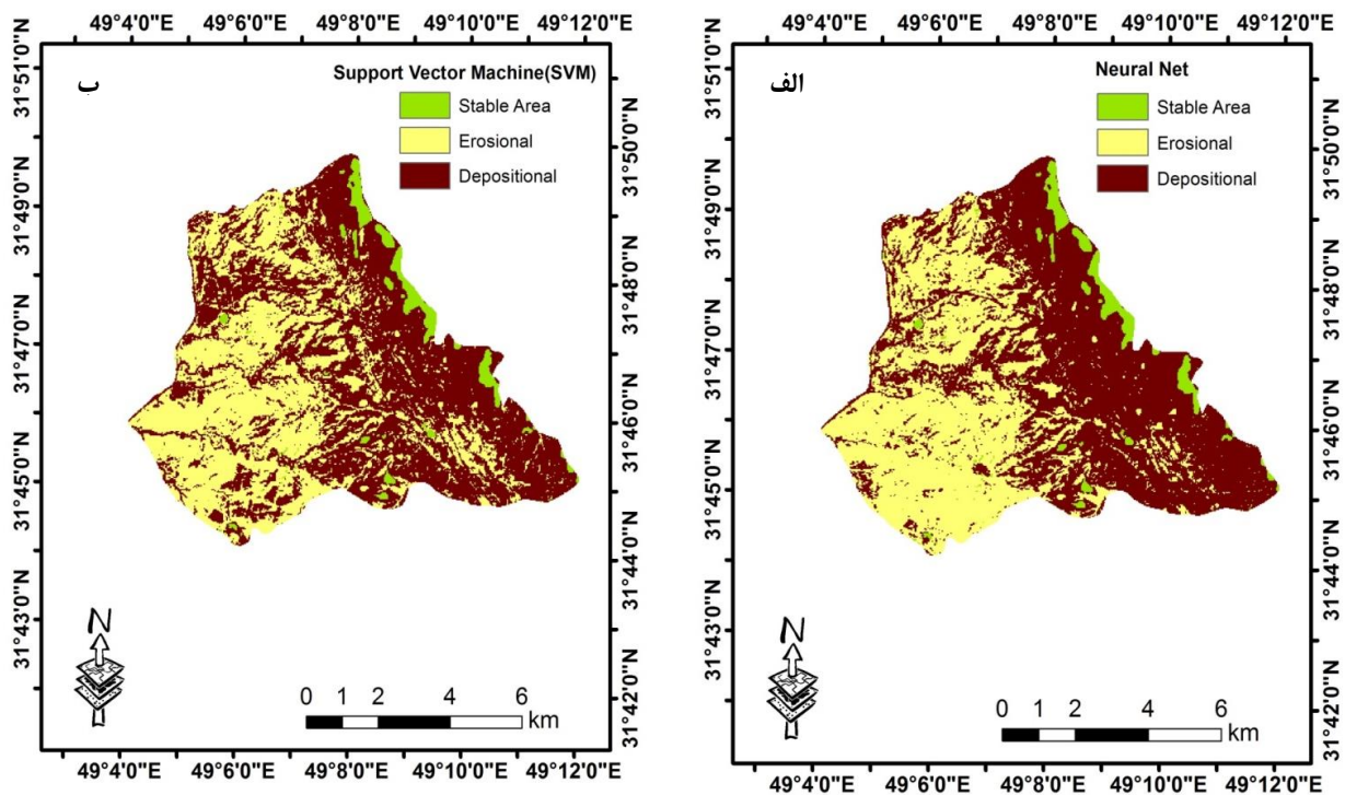
شکل ۹- نقشه‌ی تفکیک سطوح فرسایشی و رسوبی با استفاده از الگوریتم‌های شبکه عصبی (الف) و ماشین بردار پشتیبان (ب) در تلفیق با شاخص‌های سنجش از دور
