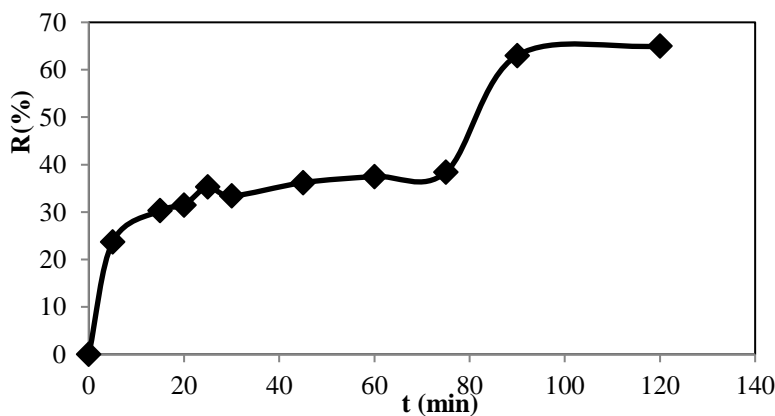
شکل ۲. اثر زمان بر راندمان جذب رنگ (غلظت اولیه جذب شونده: ۱۰ mg/L، وزن جاذب: ۱ g، pH= ۱۲)
