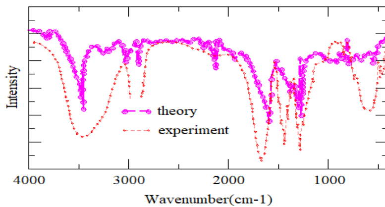
شکل ۱۱. طیف IR تجربی با داده‌های نظری
