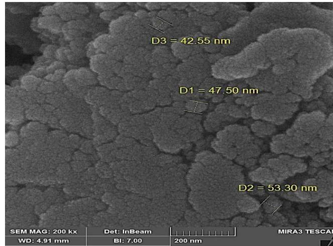
شکل ۷. تصویر SEM جاذب
