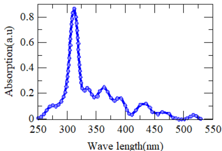
شکل ۱۲. طیف جذب اپتیکی ساختار A
